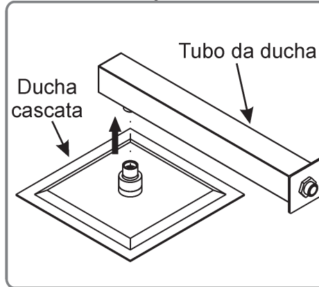
2° PASSO - Montar a ducha cascata no tubo.
