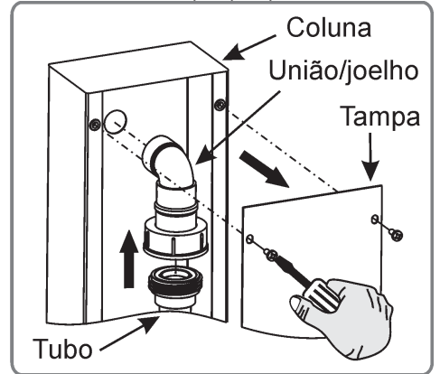
3° PASSO - Abrir a tampa da coluna e retire a união/jelho do tubo.
