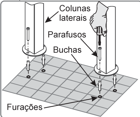
10° PASSO - Marcar, fazer as furações e inserir as buchas. Depois fixe as colunas laterais com os parafusos.
