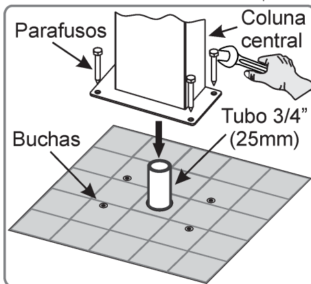
7° PASSO - Encaixe a coluna central no tubo de espera e fixe com os parafusos.
