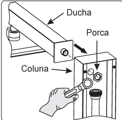
4° PASSO - Fixar a ducha na coluna central com a porca.
