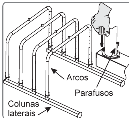
8° PASSO - Alinhe os arcos nas colunas laterais e fixe com os parafusos.
