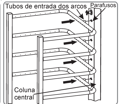
9° PASSO - Encaixe os tubos de entrada dos arcos nos furos da coluna central até os arcos encostarem nos parafusos.
