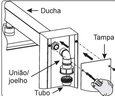
5° PASSO - Fixar a união/jelho na ducha e no tubo e feche a tampa.
