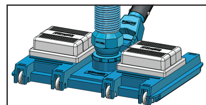
Exemplo 2: Instalação do aspirador no dispositivo de aspiração
